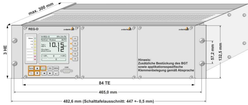
Baugruppenträger 84 TE Frontansicht - Merkmal B92/B93/B95
