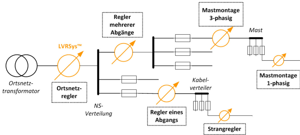
Einsatzmöglichkeiten des LVRsystm bei Netzbetreibern
