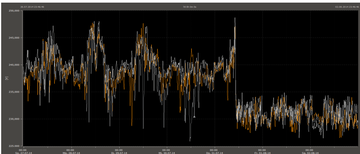
Spannungsprofil eines Netzausläufers vor und nach der Inbetriebnahme LVRsyst TM
