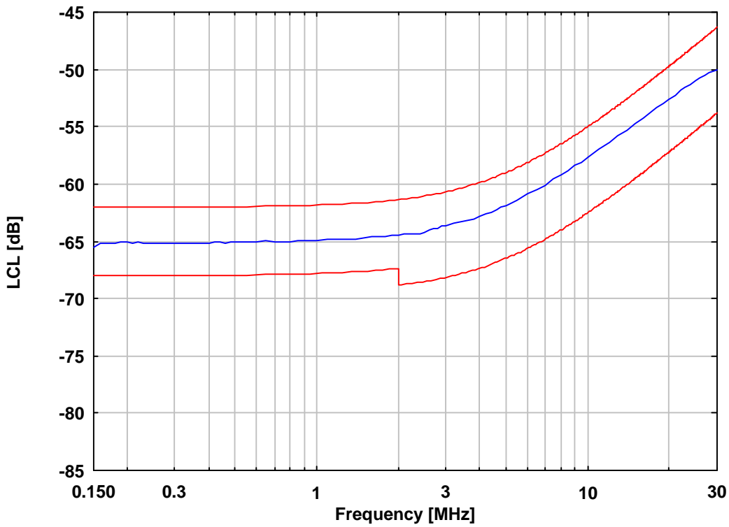
Abb. 4 Longitudinal Conversion Loss (LCL)
