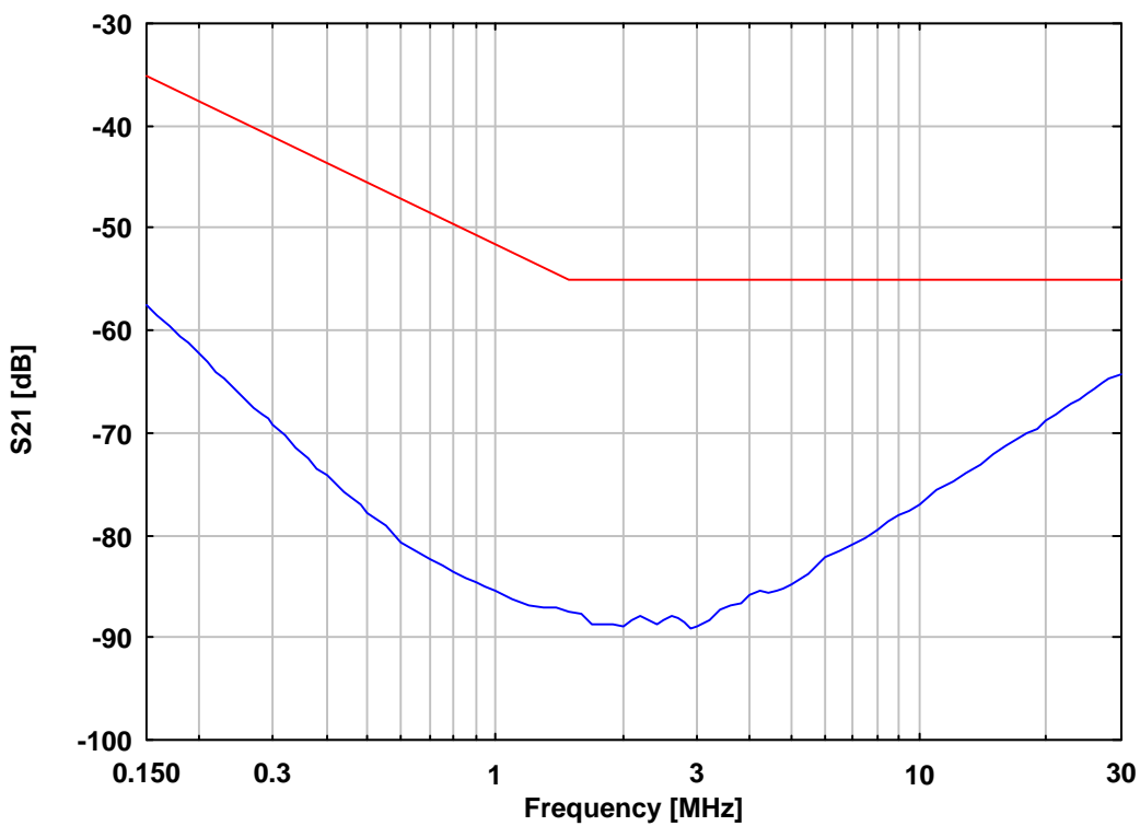
Abb. 3 Entkopplung/ Decoupling AE - EuT
